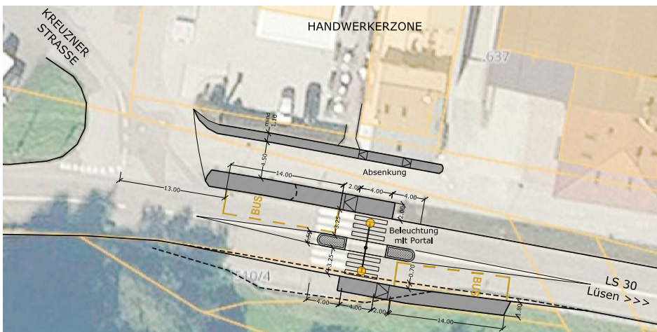
Zur Erhöhung der Sicherheit bei der Abzweigung Kreuz sind verschiedene bauliche Eingriffe geplant
