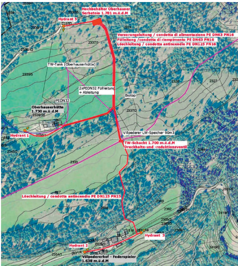
Projekt der „abgespeckten Version“: Quellsanierung, Bau eines Trink- und Löschwasserbehälters oberhalb der „Oberhauserhütte“ und Anbindungen an das Trink- und Löschwassernetz
